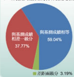
CWT成績與基測寫作成績比較
